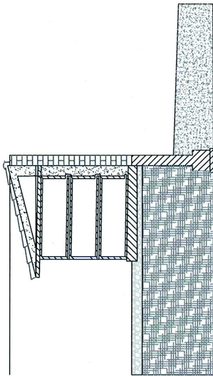
SEZIONE A-A
