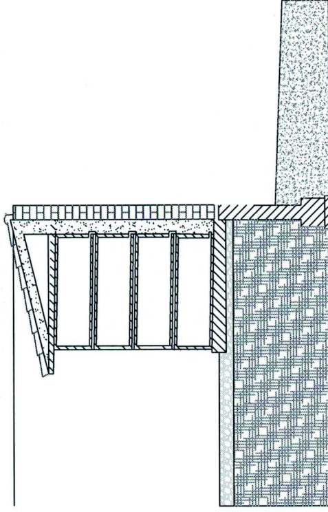
SEZIONE A-A
